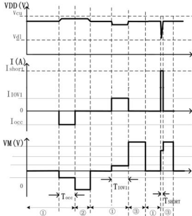
注：(1) 正常情况 (2) 过充电流状态 (3) 过放电流状态
